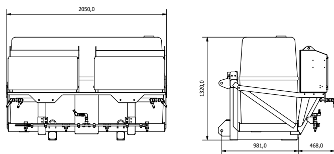
Dysspridare CLT-1.8/2.1
